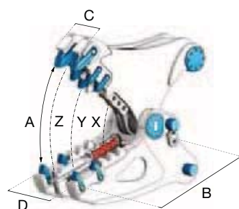
Pulverisierer / Krokodilbeißer
